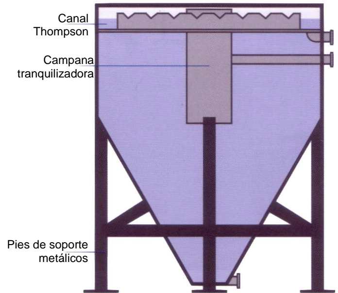
Decantador troncocónico con pies de soporte metálicos
