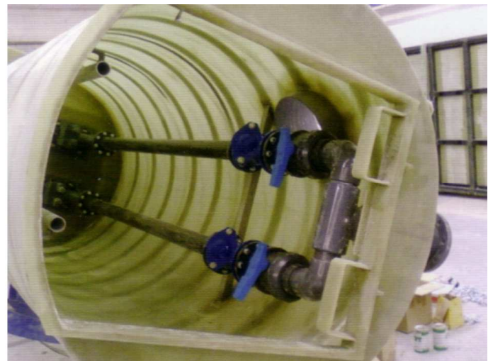
Pozo de bombeo con dos bombas sumergibles instaladas con pedestal y guías de extracción.
